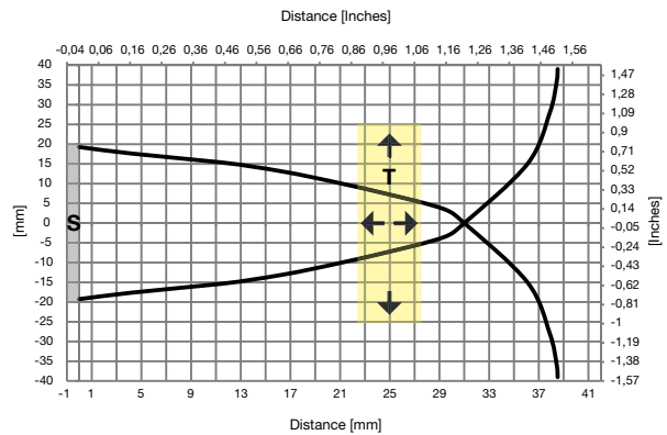
Fig. 2 Non-flush
